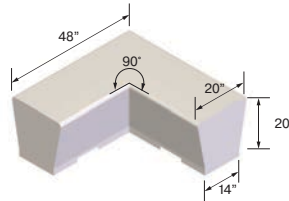
ZB.WL.04
