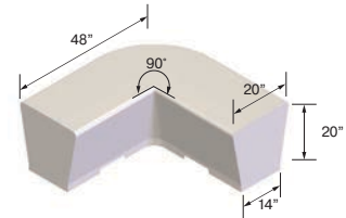
ZB.WL.05
