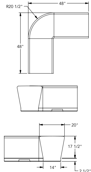
Details - ZB.WL.05
